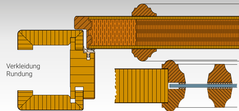
TÜRPROFILSTAMMF1
