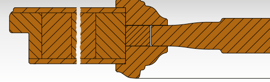
TÜRPROFILSTAMMR2
