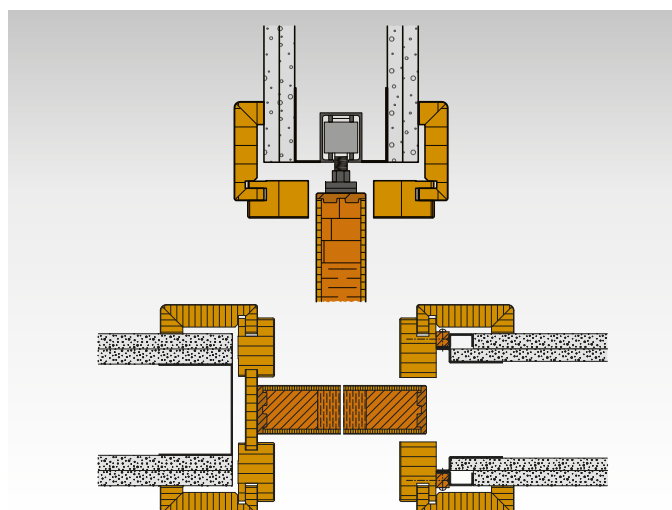
HOLZSCHIEBETÜRE
