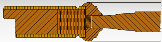
TÜRPROFILSTAMMS4
