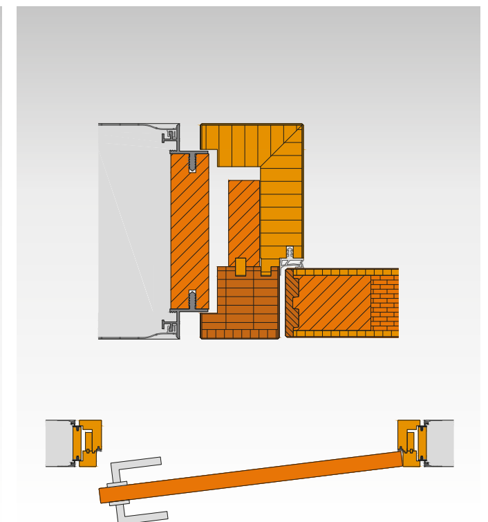
N5B1E Gehungstock wandbündig Design N5 bündig einschlagend Verkleidung Aufrecht Anschluss mit Blindstock
