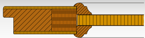
TÜRPROFILSTAMMS2
