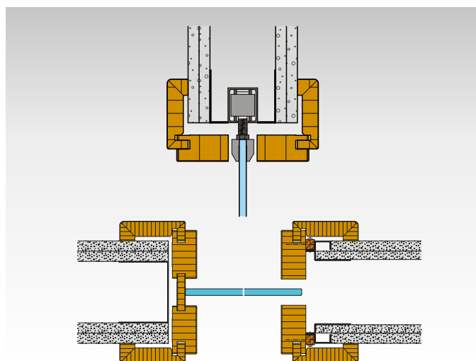
GANZGLASSCHIEBETÜRE
