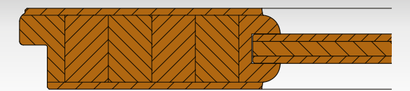
TÜRPROFILSTAMME2
