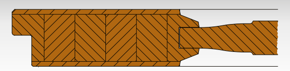
TÜRPROFILSTAMMK6
