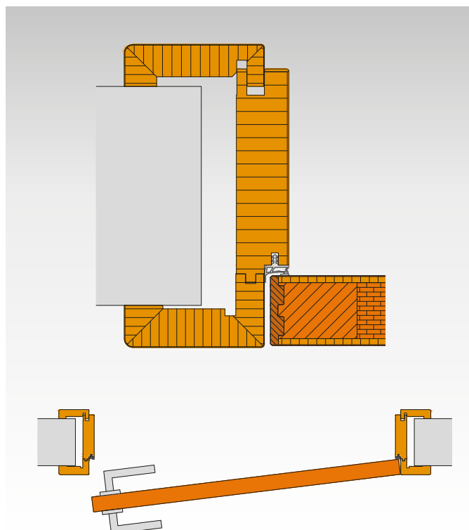
FB1E Futterstock Design F bündig einschlagend Verkleidung Rundung, 80 mm
