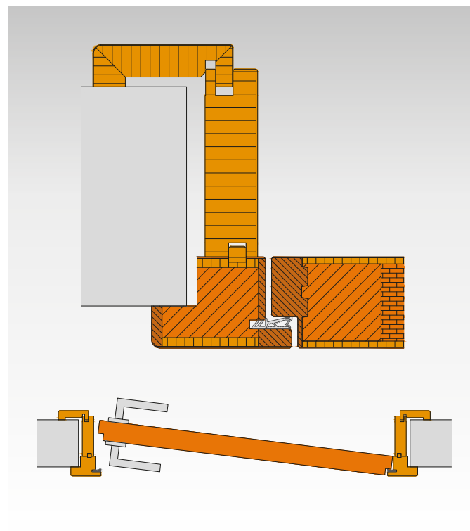
FR1 Futterstock Design F Return – Türblatt in Laibung öffnend Verkleidung Rundung, 80 mm
