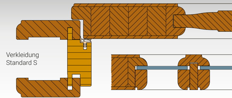
TÜRPROFILSTAMMK1
