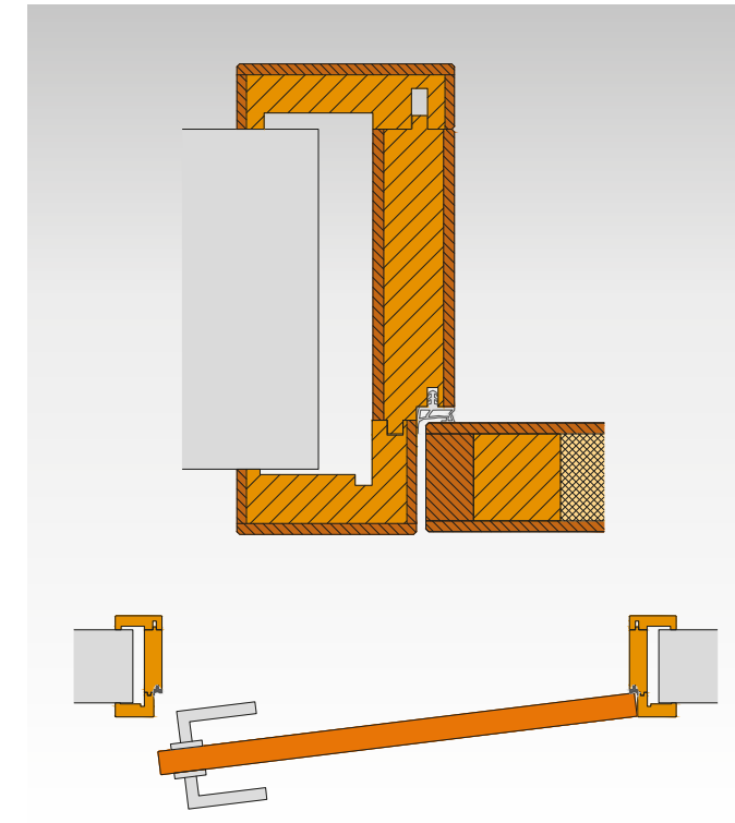
F4B1E Blockfutterstock Design F4 bündig einschlagend Verkleidung Aufrecht
