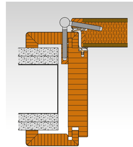
FUTTERSTOCK FF2E FUTTERSTOCK DESIGN F Falz: F2E Türstärke: 44 mm Klimaklasse: b-c RW-Wert: 32–37dB (Schalldichte)
