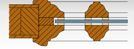
TÜRPROFILSTAMMK6
