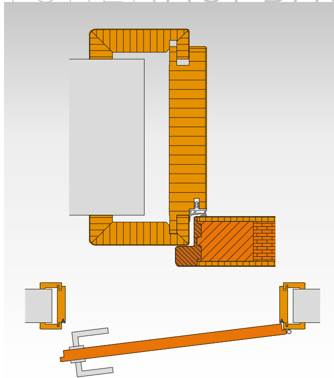
FF1 Futterstock Design F Türblatt überfälzt Verkleidung Rundung, 80 mm
