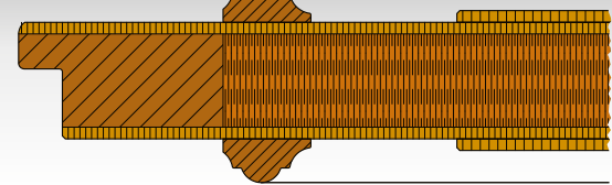
TÜRPROFILSTAMMS5
