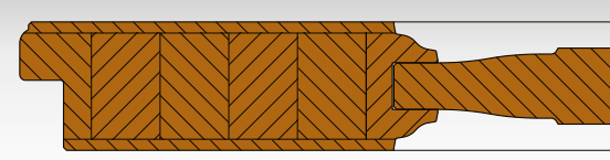
TÜRPROFILSTAMMK2
