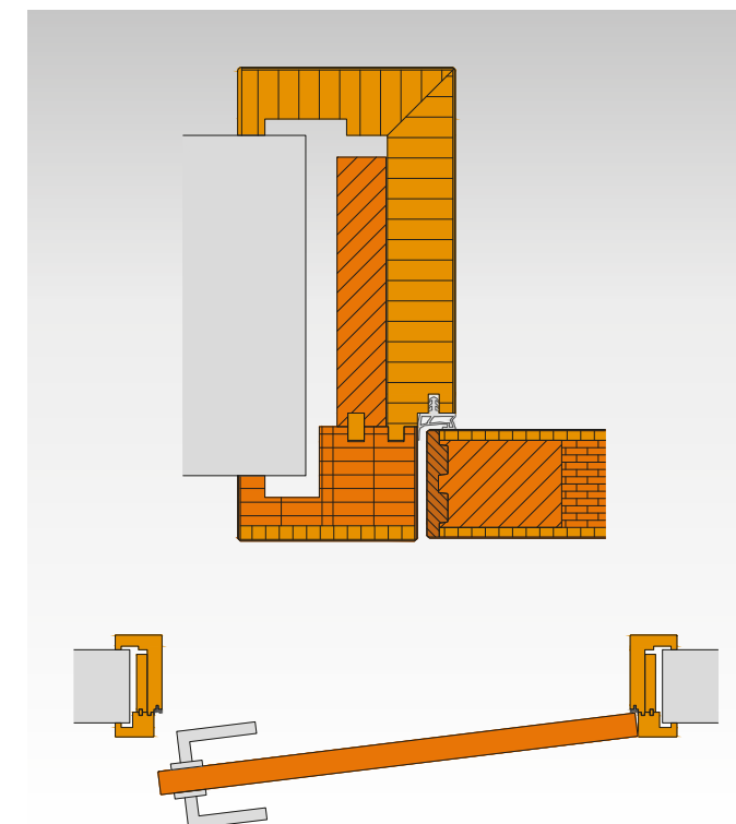
F3B1E Gehungstock Design F3 bündig einschlagend Verkleidung Aufrecht
