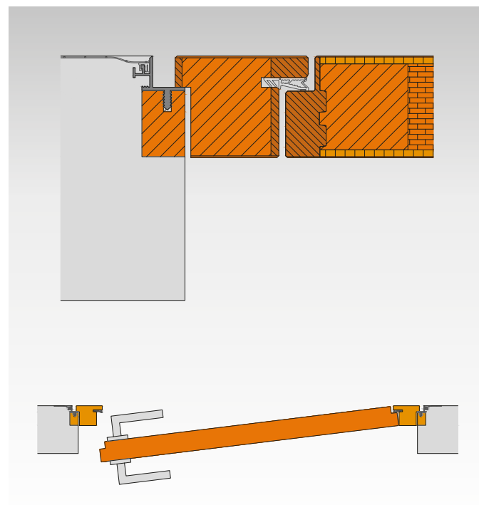
PB2E Pfosten beidseitig flächenbündig Anschluss wandbündig mit Blindstock
