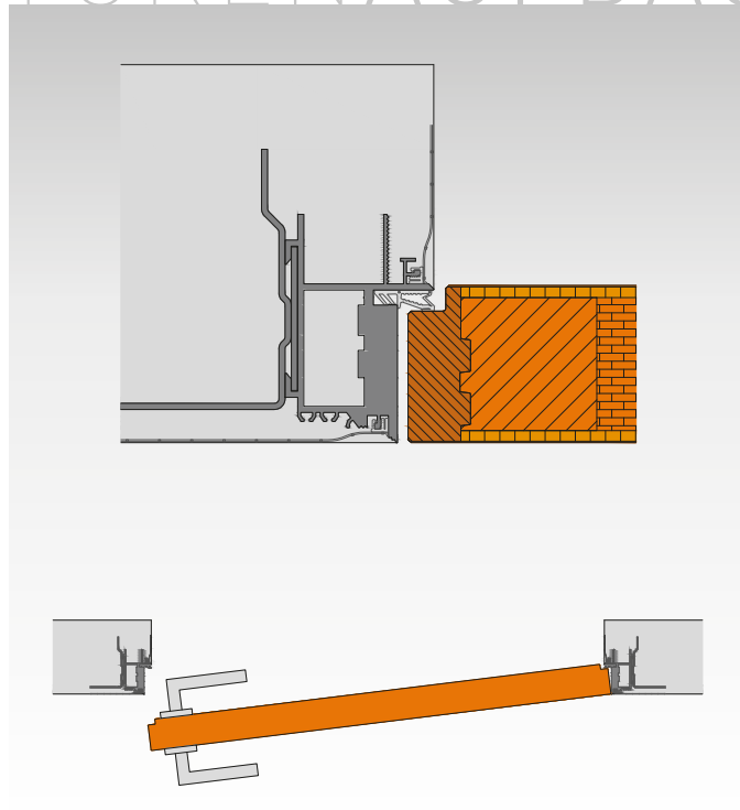
UB5 System rahmenlos Öffnung Profilseite Türblatt wandbündig
