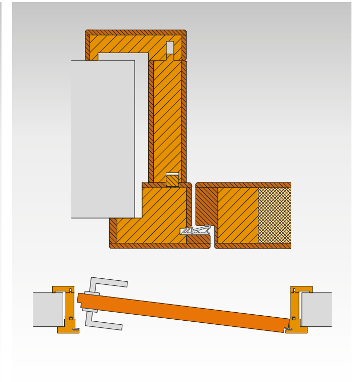
F4R1 Blockfutterstock Design F4 Return – Türblatt in Laibung öffnend Verkleidung Aufrecht
