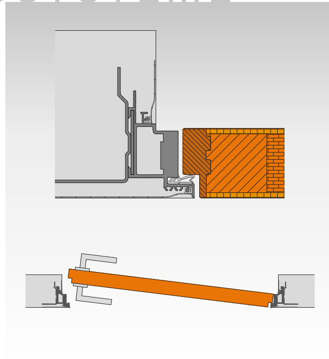
UR6 System rahmenlos Öffnung Laibungsseite Türblatt wandbündig
