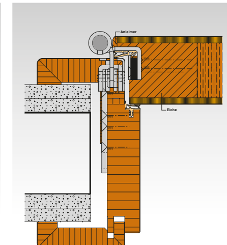
FUTTERSTOCK FF2T FUTTERSTOCK DESIGN F Falz: F2T Türstärke: 62 mm Klimaklasse: b-c RW-Wert: 32–42dB (Schalldichte) U-Wert: 1,44 – 0,97 W/m²K
